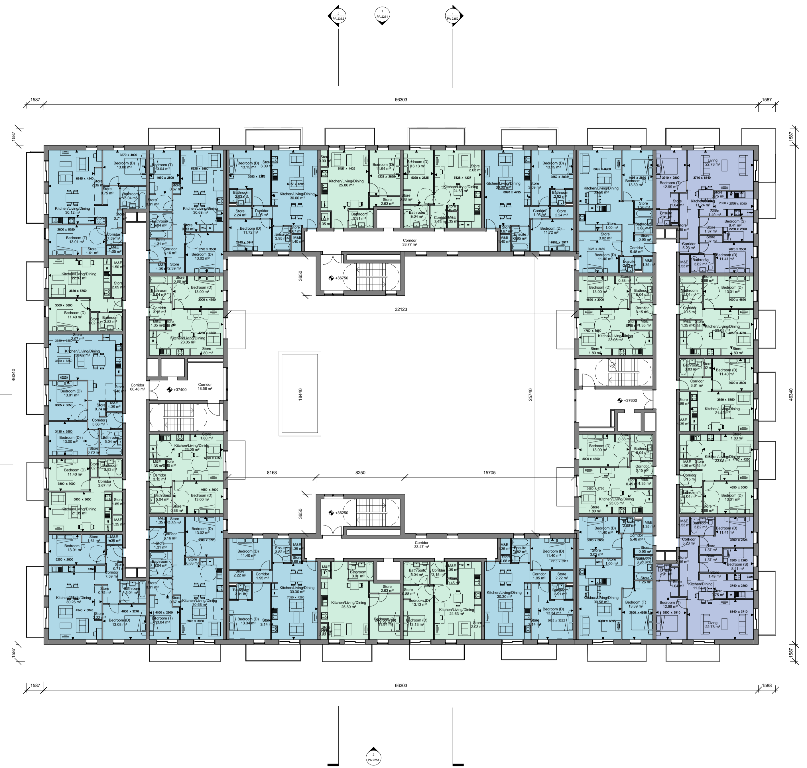
2 Block E - Level 03 1 : 200
