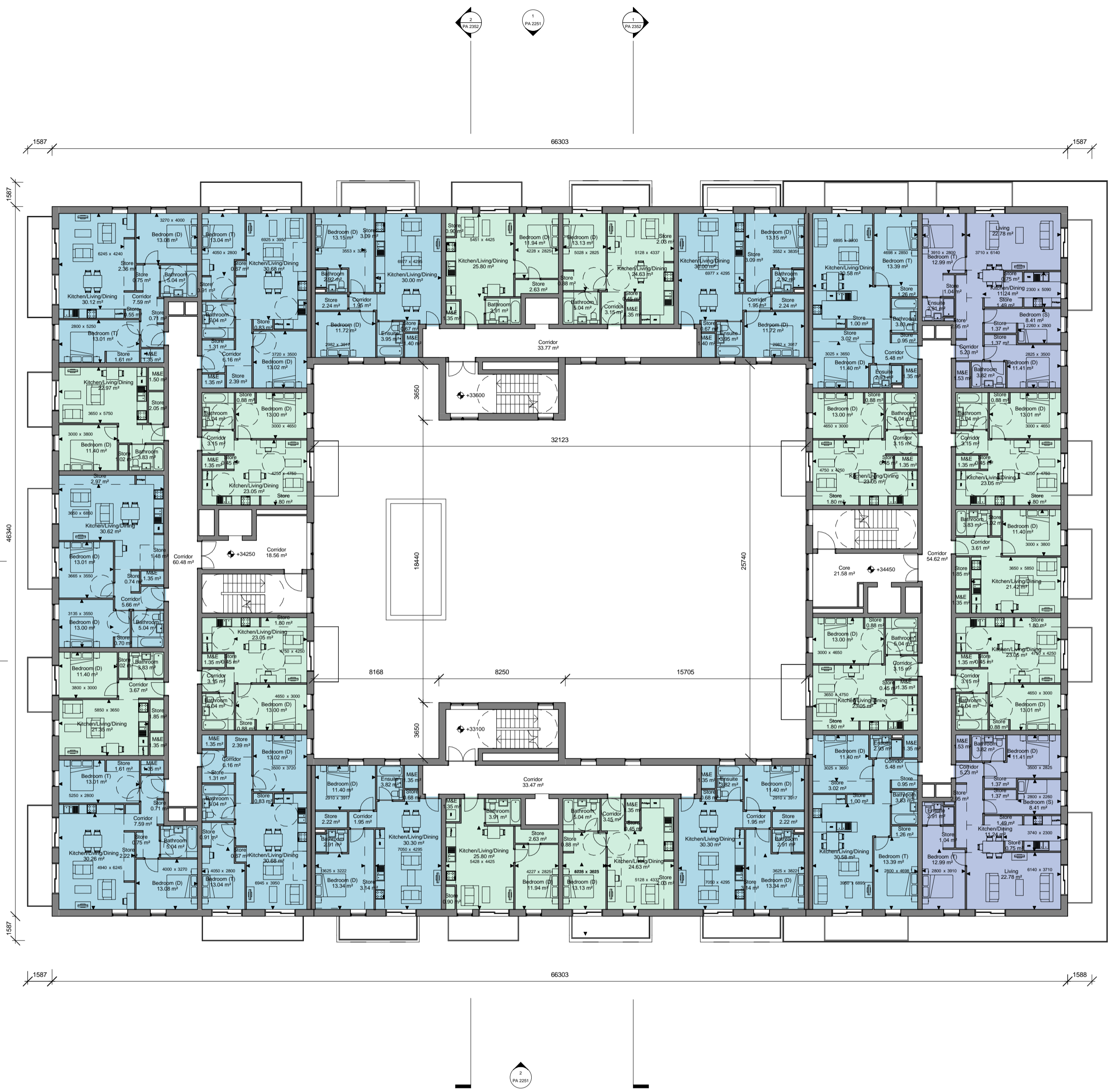
1 Block E - Level 02 1 : 200
