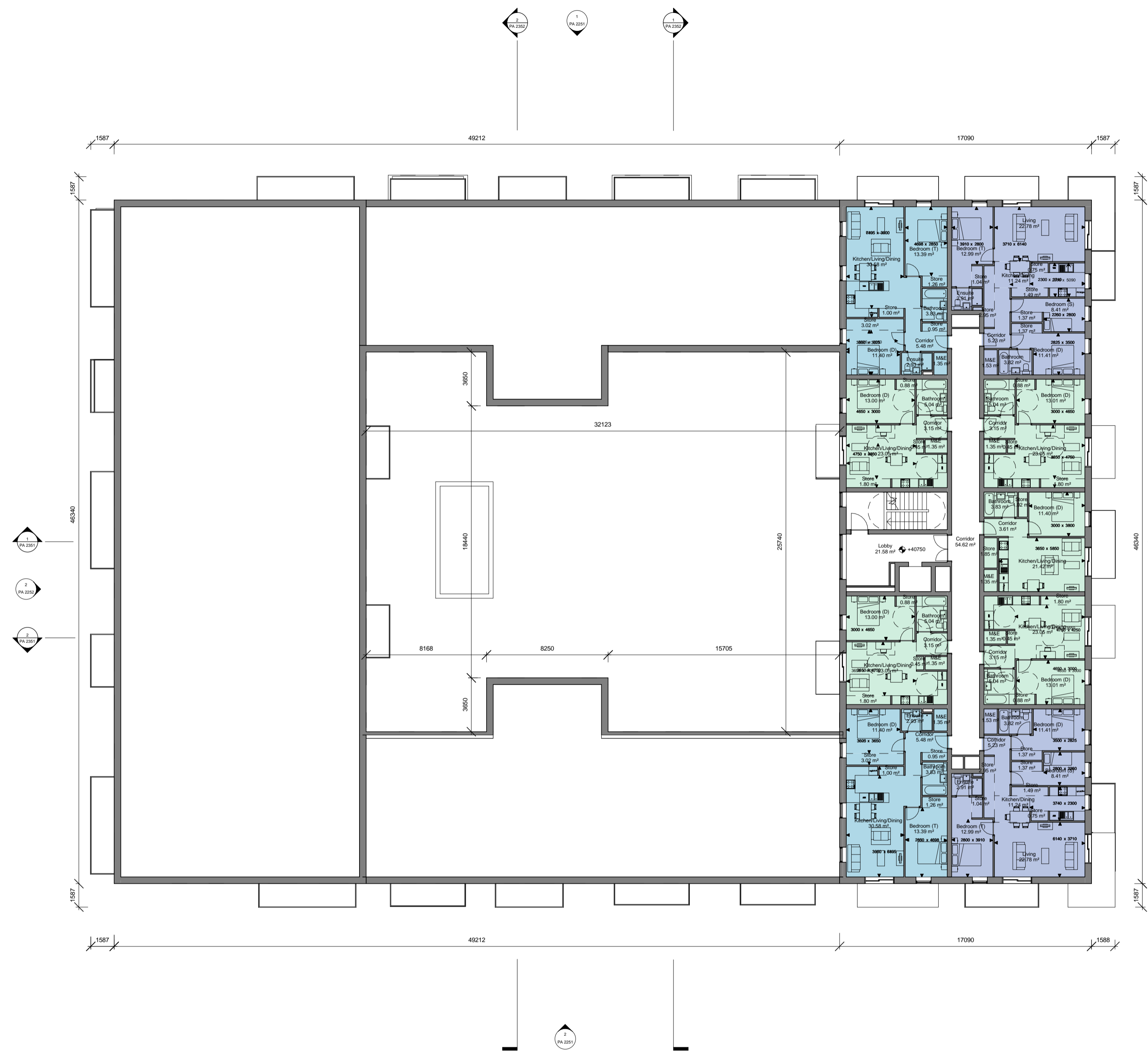
1 Block E - Level 04 1 : 200
