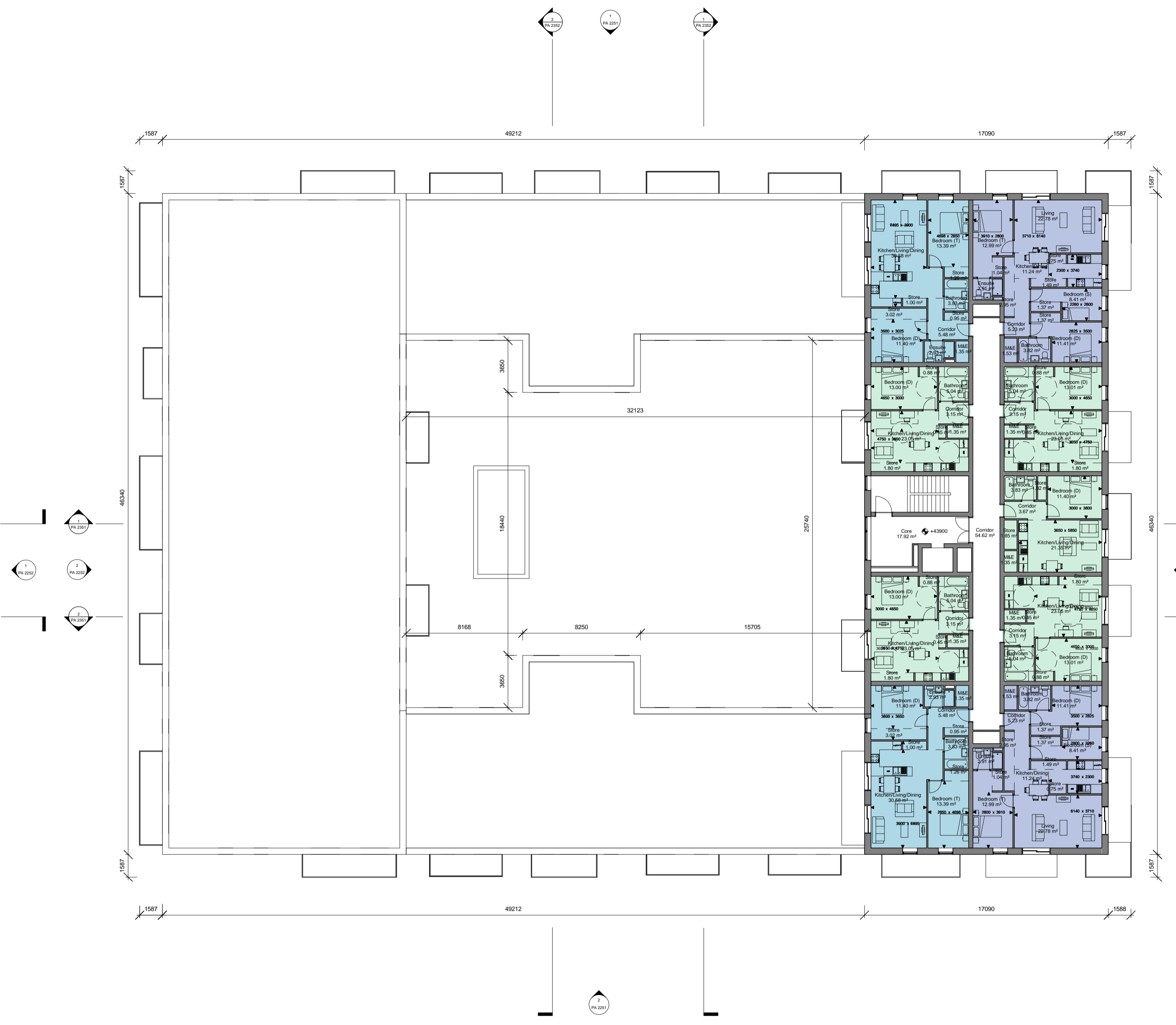
2 Block E - Level 05 1 : 200
