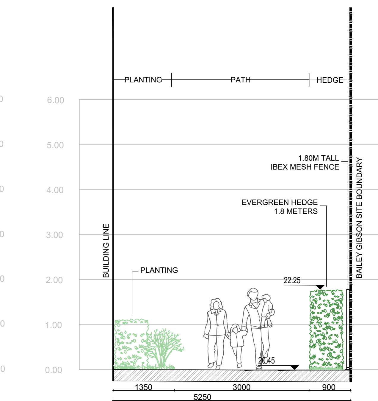
03 SECTION 03 SCALE: 1:50 @ A1
