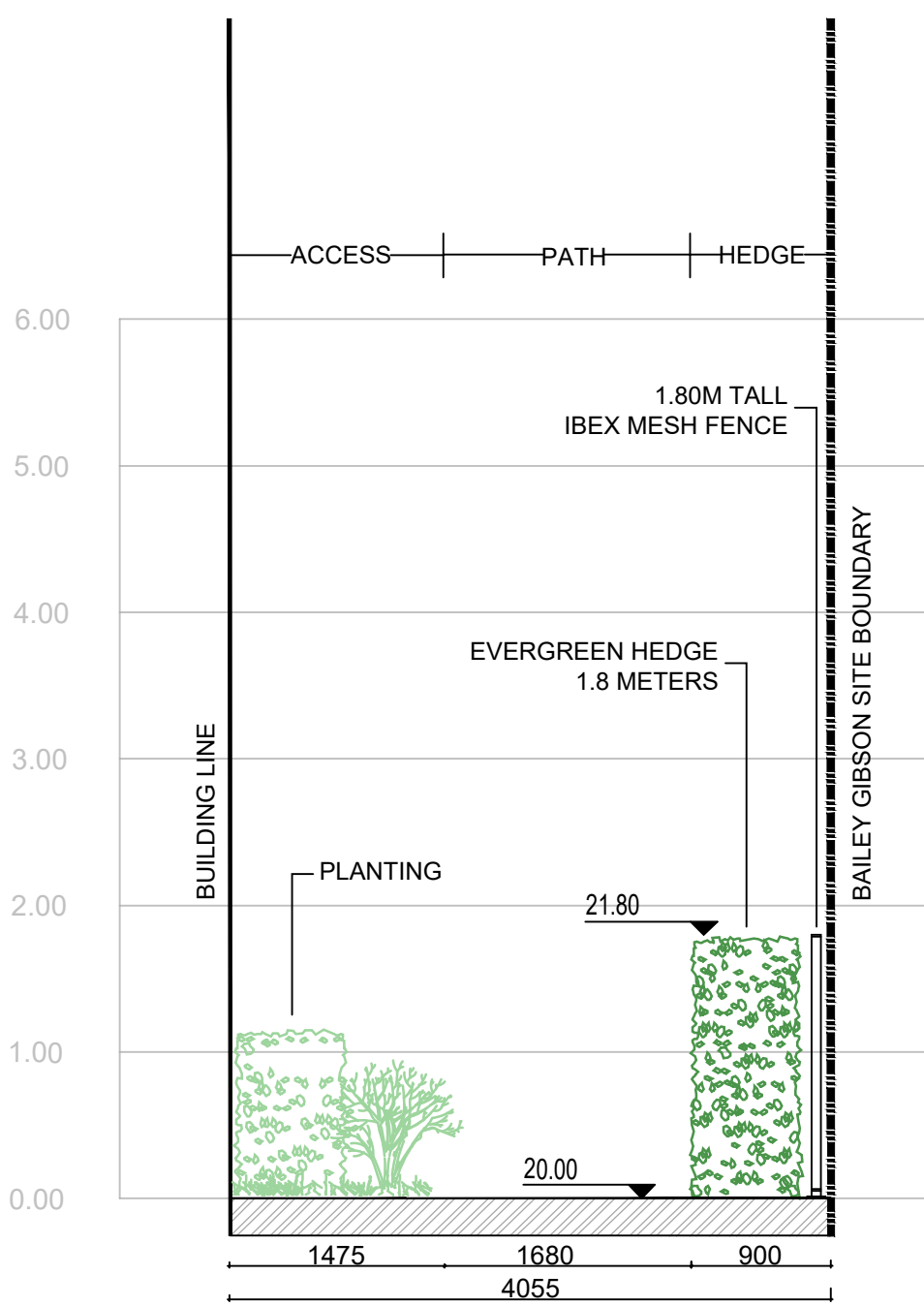
05 SECTION 05 SCALE: 1:50 @ A1
