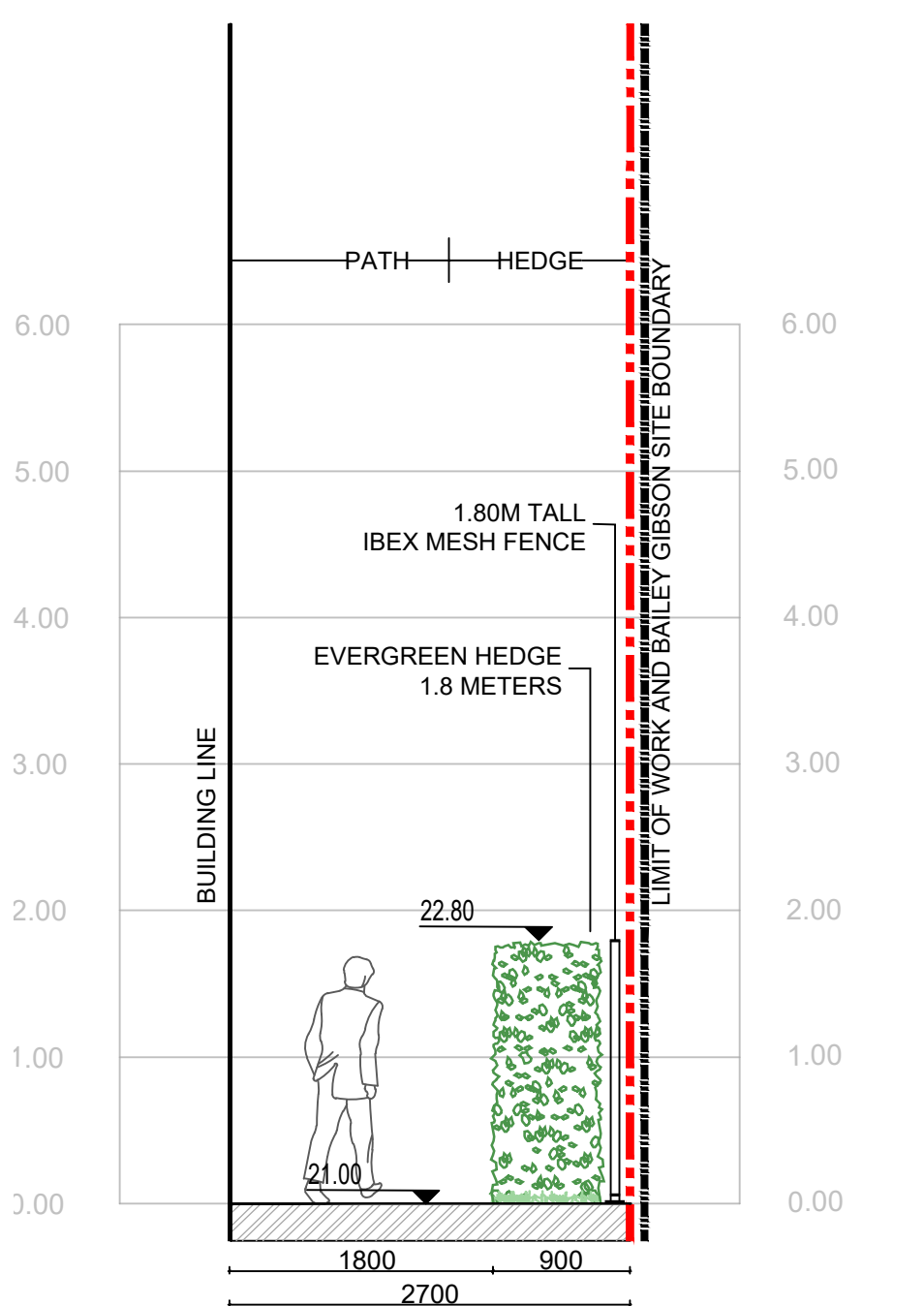
01 SECTION 01 SCALE: 1:50 @ A1
