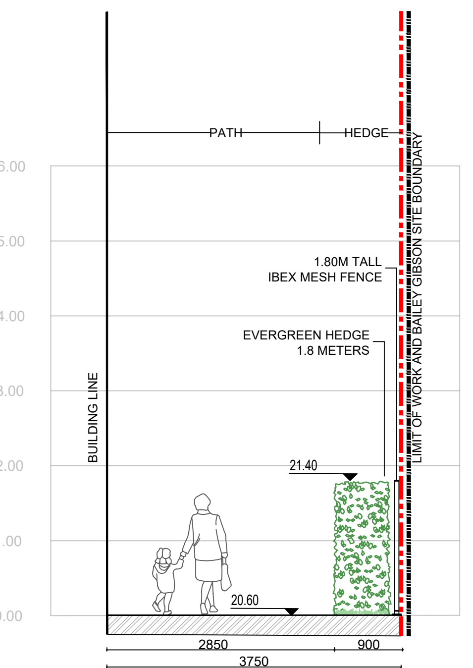
02 SECTION 02 SCALE: 1:50 @ A1
