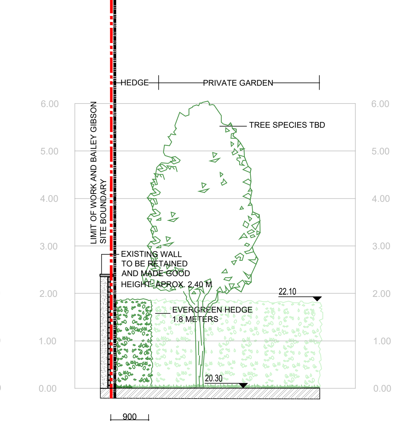
08 SECTION 08 SCALE: 1:50 @ A1
