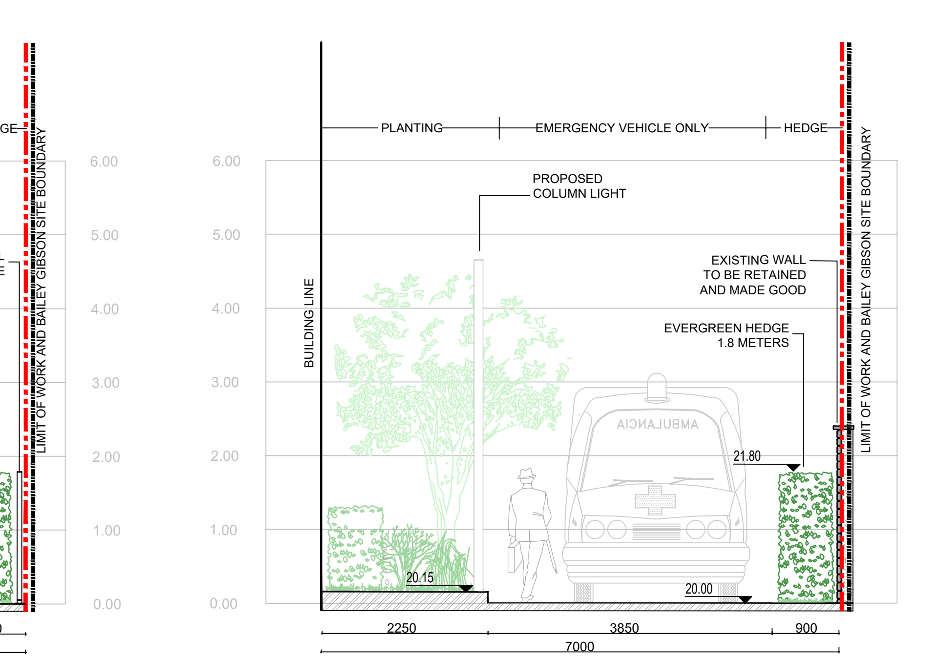
07 SECTION 07 SCALE: 1:50 @ A1
