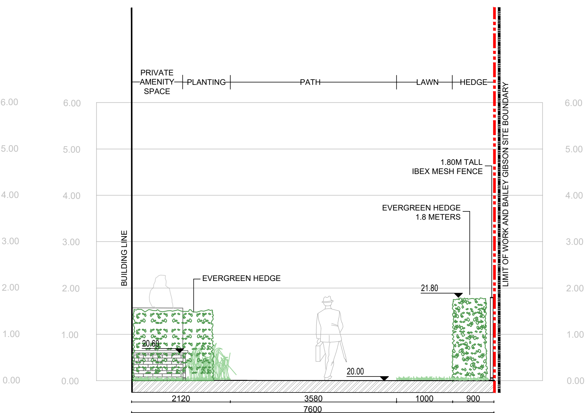
04 SECTION 04 SCALE: 1:50 @ A1
