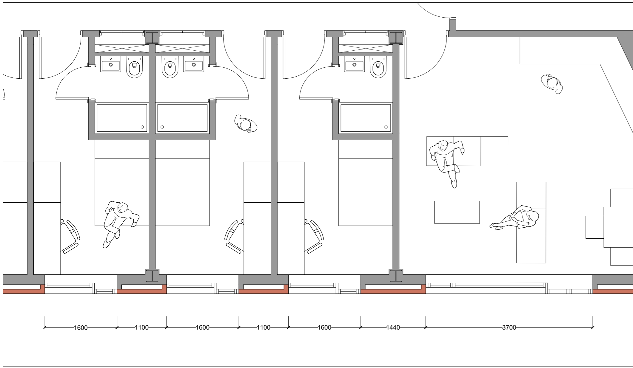
PLAN: 1:50
